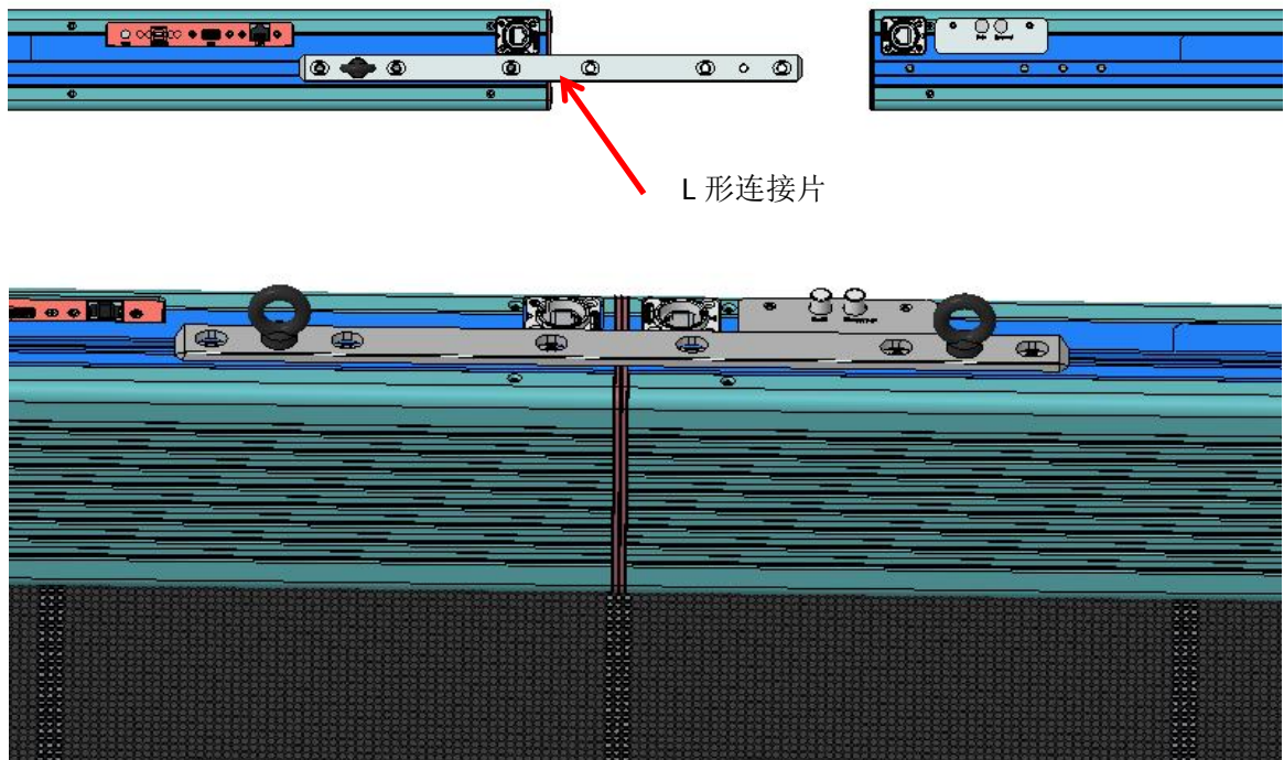
图 3-2 拼接导轨条
