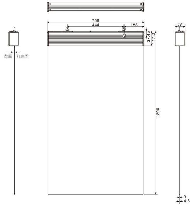
图 1-1 55"整机吊装
