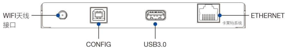
图 2-2 卡莱特控制器外置接口详解
