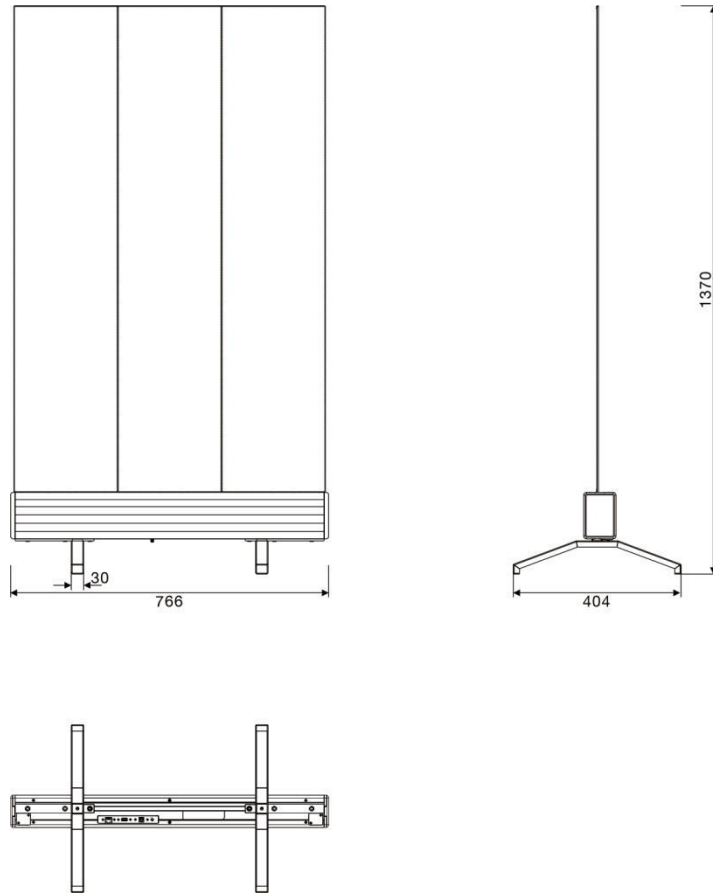
图 1-3 55"整机立式
