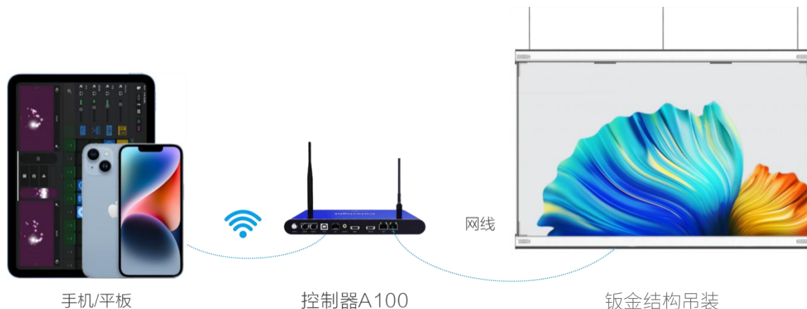
附录图 1-6 异步控制系统示意图
