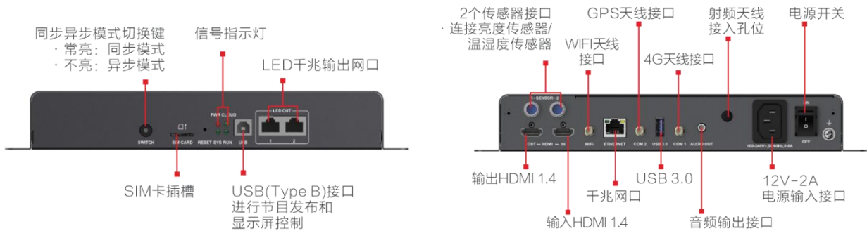
附录图 1-2 诺瓦控制盒·前面板（左图），后面板（右图）
