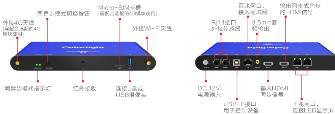
附录图 1-3 卡莱特控制盒·前面板（左图），后面板（右图）
