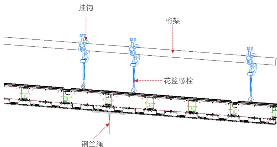
图 2-2 上梁安装图
