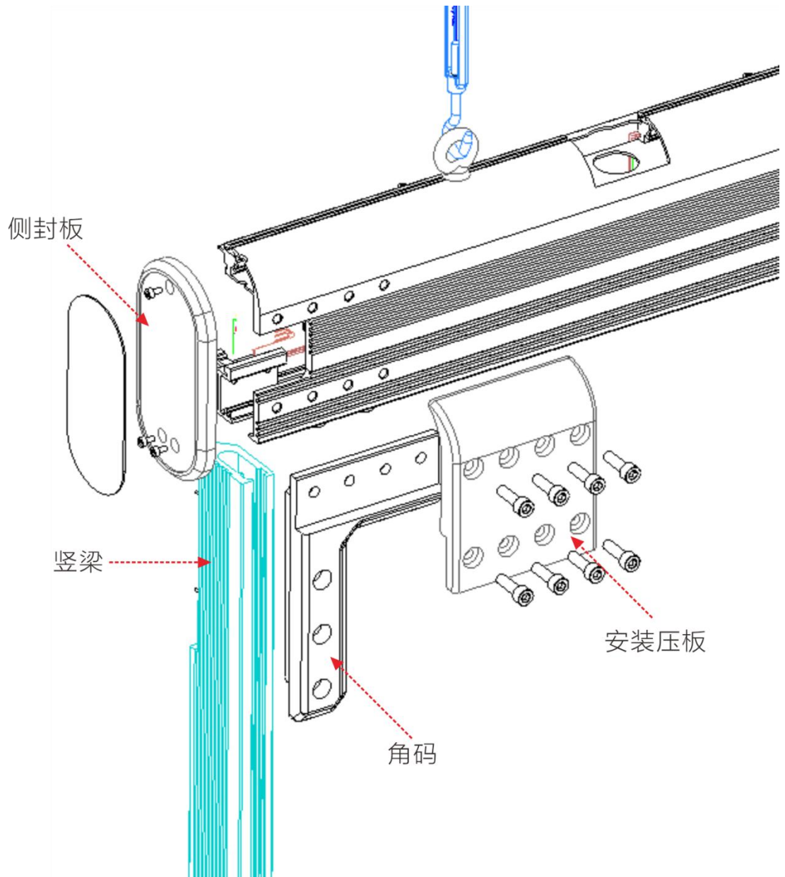
图 2-3 竖梁安装图
