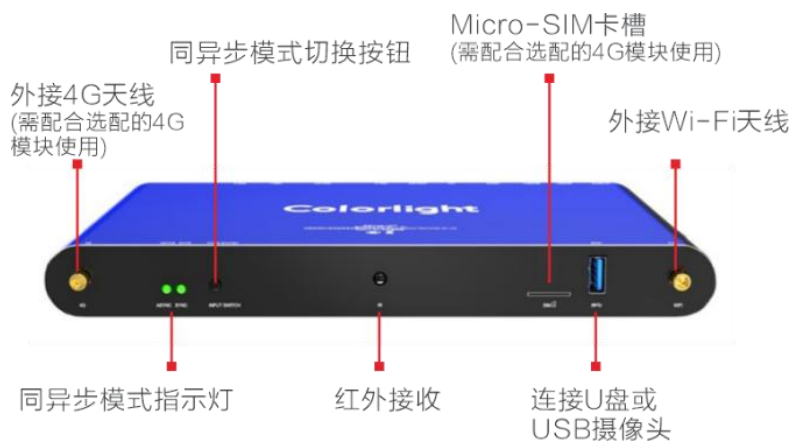
附录图 1-1 系统配件图
